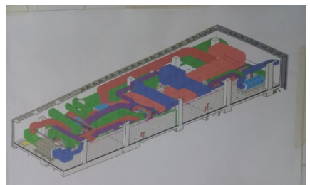
Tour BCP à Casablanca city financier: Fourniture et pose des jackettage en alu des gaines rectangulaires du local technique CTA- Client Ventec Maroc
